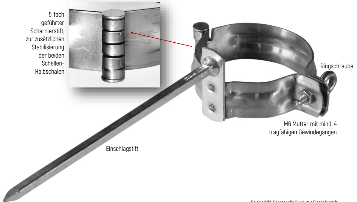
Beispielbild: Rohrschelle Rund, mit Einschlagstift
